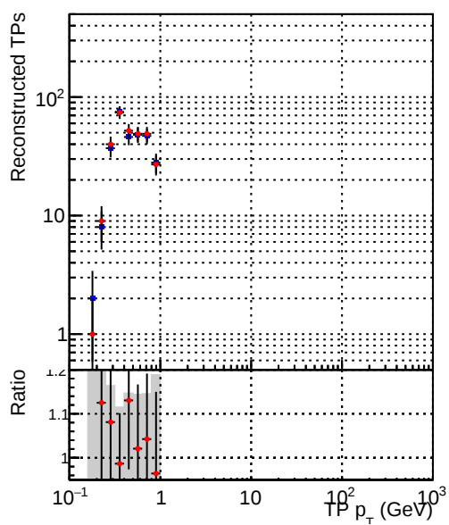
—•— DQM_CKF_TTbase —•— DQM_CKF_TT_retrainOldFiles125_v2_prelimWP_epoch4
