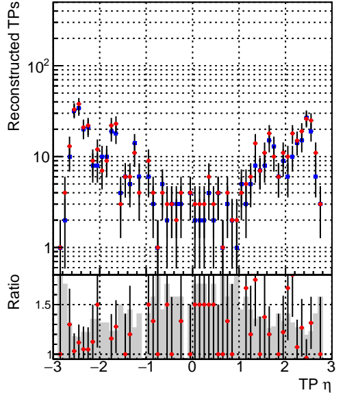
■ DQM_CKF_TTbase ■ DQM_CKF_TT_retrainOldFiles125_v2_prelimWP_epoch4
