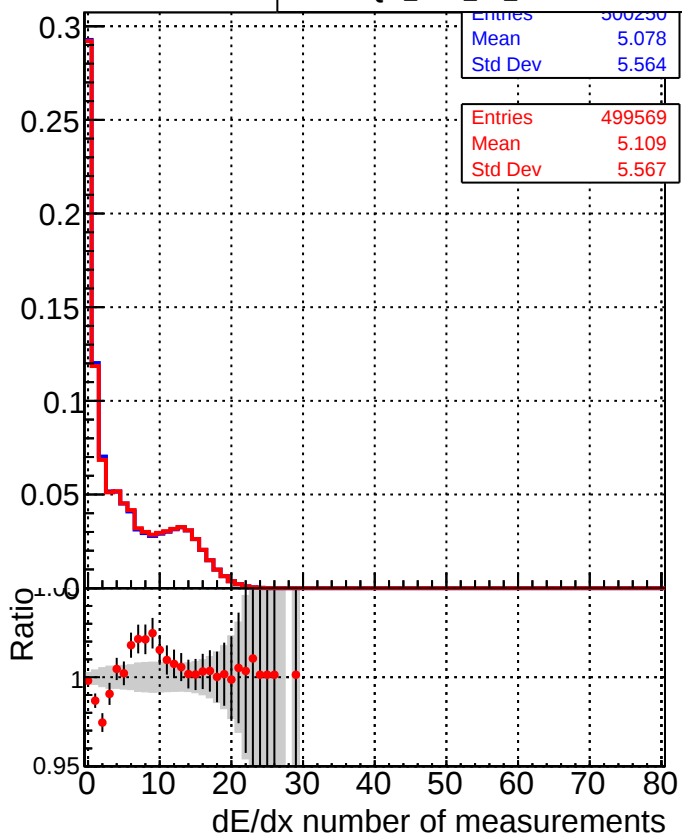
■ DQM_CKF_TTbase ● DQM_CKF_TT_retrainOldFiles125_v2_prelimWP_epoch4
