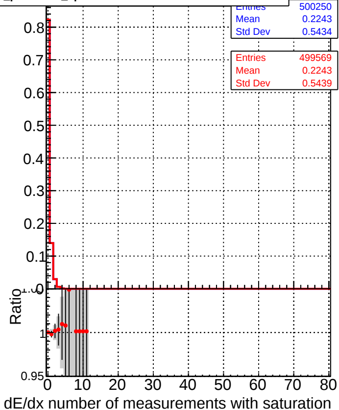
■ DQM_CKF_TTbase ● DQM_CKF_TT_retrainOldFiles125_v2_prelimWP_epoch4
