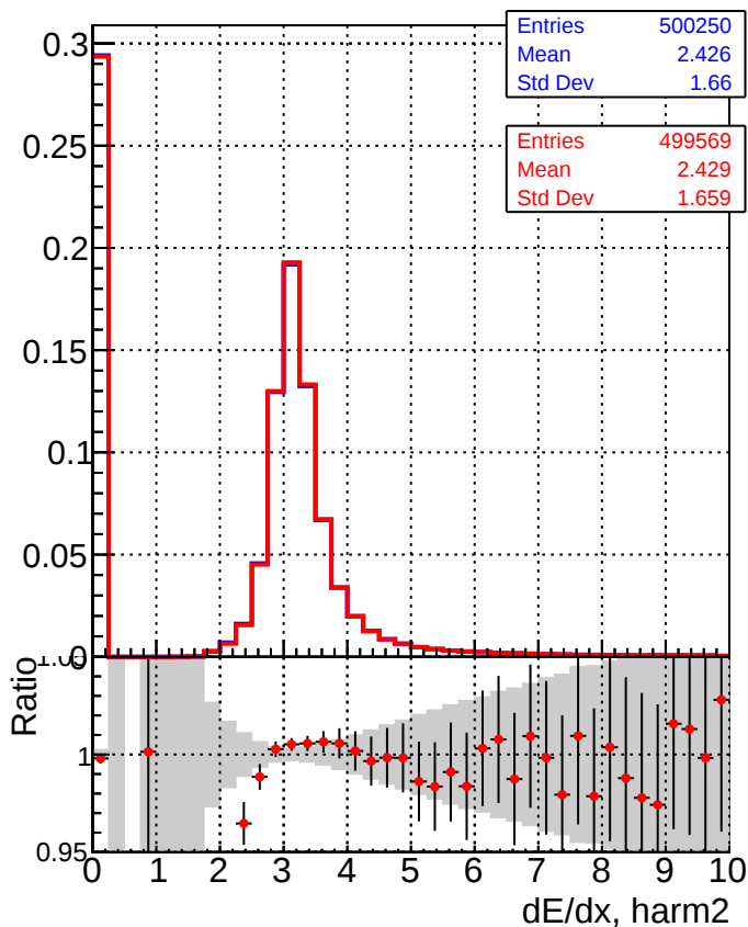
■ DQM_CKF_TTbase ● DQM_CKF_TT_retrainOldFiles125_v2_prelimWP_epoch4
