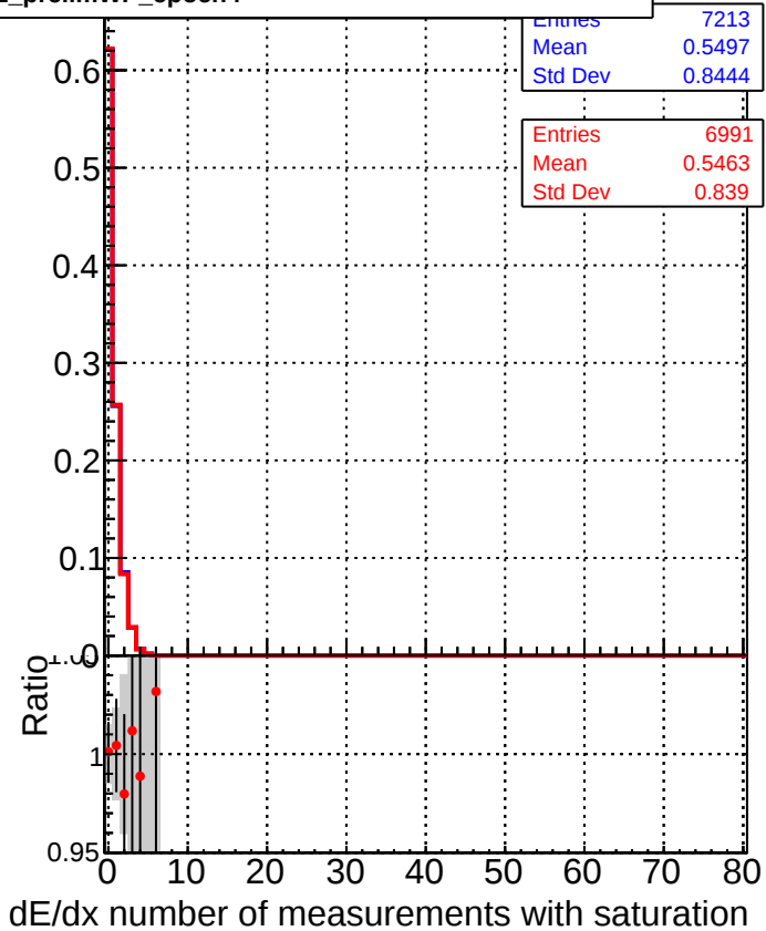
DQM_CKF_TTbase DQM_CKF_TT_retrainOldFiles125_v2_prelimWP_epoch4
