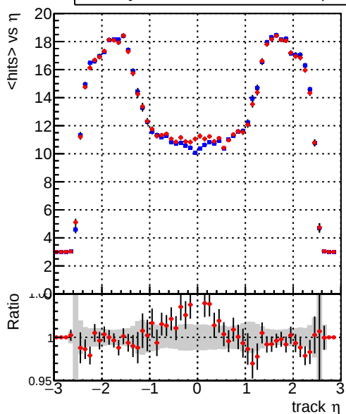
— DQM_CKF_TTbase — DQM_CKF_TT_retrainOldFiles125_v2_prelimWP_epoch4 mean hits
