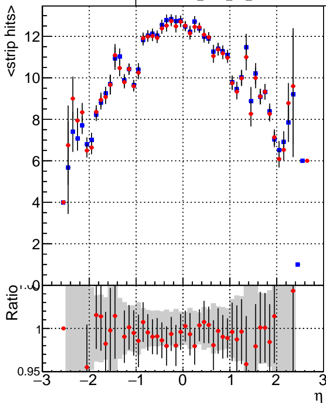
■ DQM_CKF_TTbase ● DQM_CKF_TT_retrainOldFiles125_v2_prelimWP_epoch4
