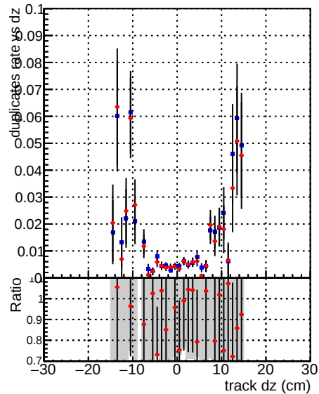
—●— DQM_CKF_TTbase —●— DQM_CKF_TT_retrainOldFiles125_v2_prelimWP_epoch4
