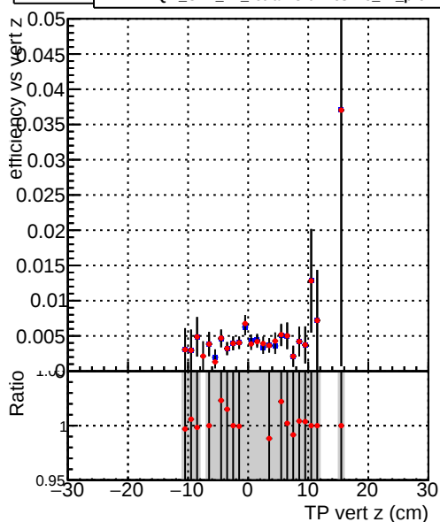
Efficiency — DQM_CKF_TT_retrainOldFiles125_v2_prelimWP_epoch4
