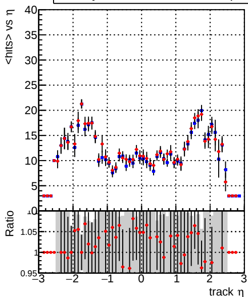
mean hits — DQM_CKF_TTbase — DQM_CKF_TT_retrainOldFiles125_v2_prelimWP_epoch4
