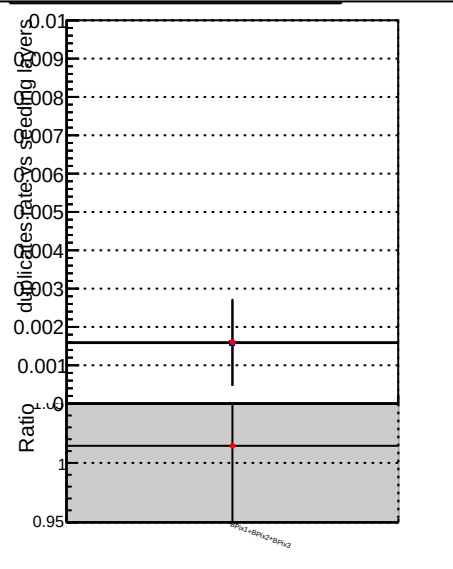
\blacksquare (blue) DQM CKF TTbase \bullet (red) DQM CKF TT_retrainOldFiles125_v2_prelimWP_epoch4
