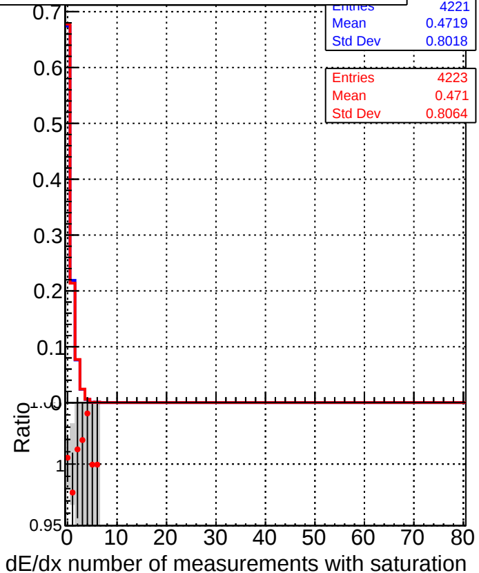
■ DQM_CKF_TTbase ● DQM_CKF_TT_retrainOldFiles125_v2_prelimWP_epoch4
