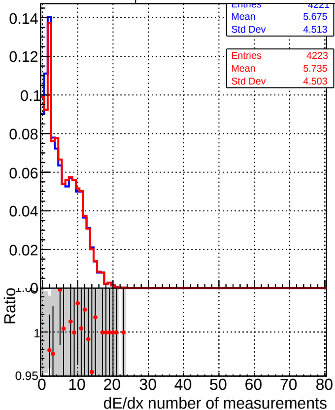
■ DQM_CKF_TTbase ● DQM_CKF_TT_retrainOldFiles125_v2_prelimWP_epoch4
