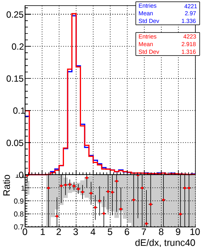
■ DQM_CKF_TTbase ● DQM_CKF_TT_retrainOldFiles125_v2_prelimWP_epoch4
