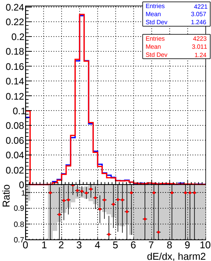
■ DQM_CKF_TTbase ● DQM_CKF_TT_retrainOldFiles125_v2_prelimWP_epoch4
