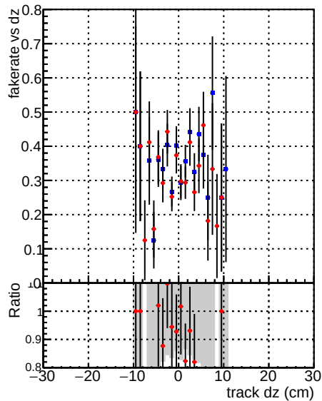
—•— DQM CKF TTbase —•— DQM CKF TT_retrainOldFiles125_v2_prelimWP_epoch4 Fake rate vs dz
