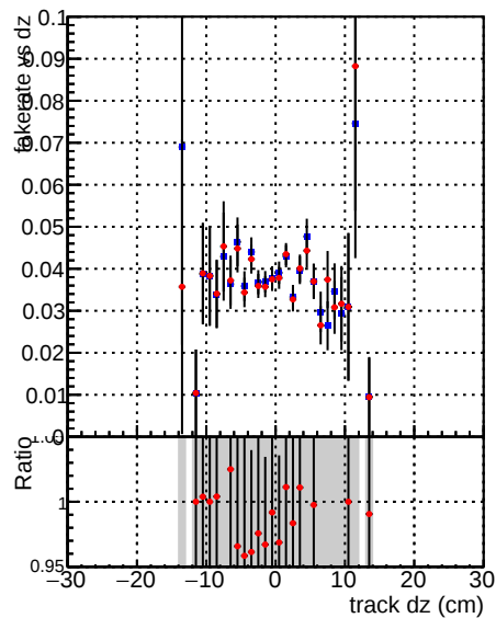
—●— DQM_CKF_TTbase —●— DQM_CKF_TT_retrainOldFiles125_v2_prelimWP_epoch4
