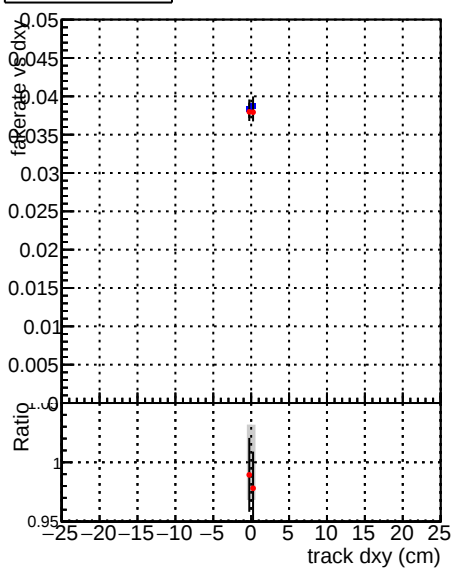
—●— DQM_CKF_TTbase —●— DQM_CKF_TT_retrainOldFiles125_v2_prelimWP_epoch4
