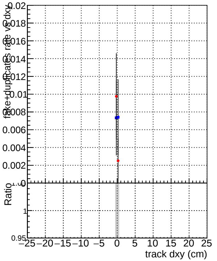
DQM_CKF_TTbase DQM_CKF_TT_retrainOldFiles125_v2_prelimWP_epoch4
