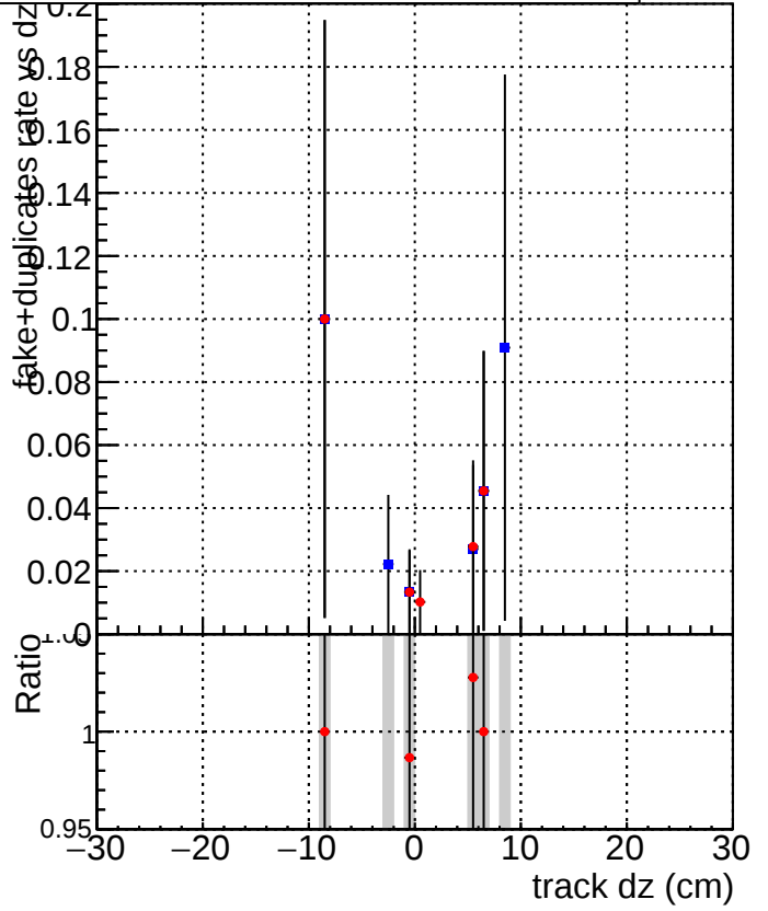
DQM_CKF_TTbase DQM_CKF_TT_retrainOldFiles125_v2_prelimWP_epoch4
