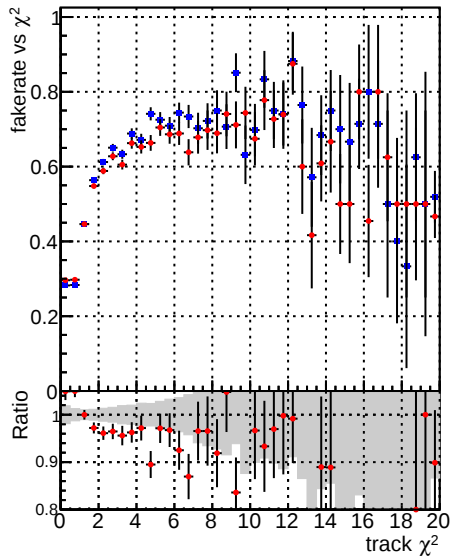
Fake rate vs. \chi^2 —◆— DQM CKF TTbase —+— DQM CKF TT_retrainOldFiles125_v2_prelimWP_epoch4
