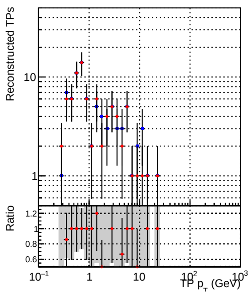
—●— DQM_CKF_TTbase —◆— DQM_CKF_TT_retrainOldFiles125_v2_prelimWP_epoch4
