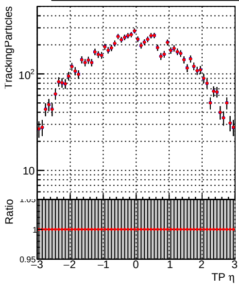
—●— DQM_CKF_TTbase —◆— DQM_CKF_TT_retrainOldFiles125_v2_prelimWP_epoch4
