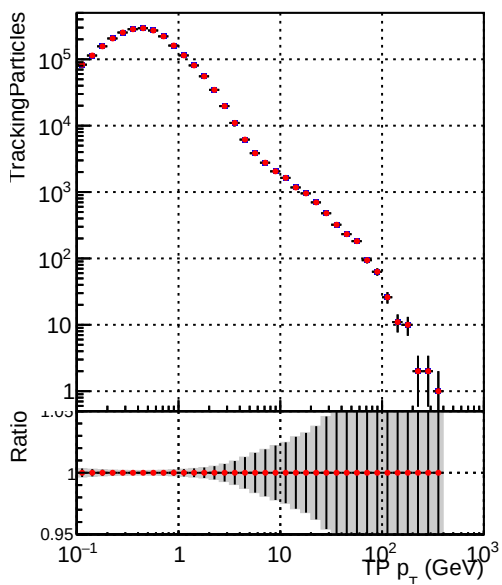
■ DQM_CKF_TTbase —●— DQM_CKF_TT_retrainOldFiles125_v2_prelimWP_epoch4
