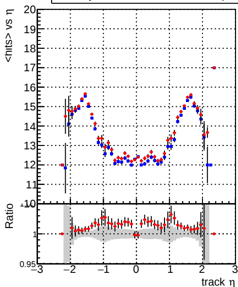
— DQM_CKF_TTbase — DQM_CKF_TT_retrainOldFiles125_v2_prelimWP_epoch4
