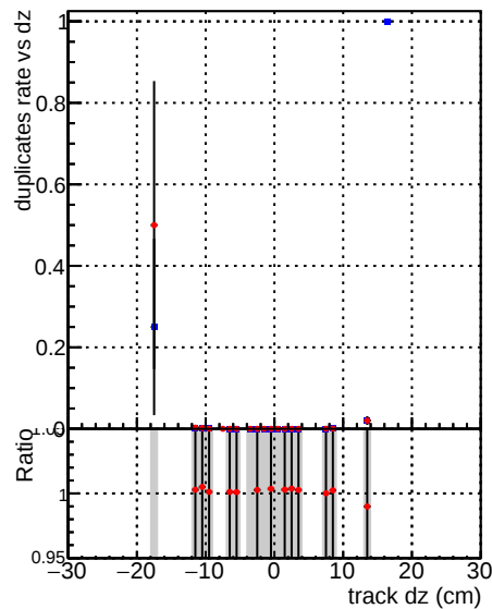
—●— DQM_CKF_TTbase —●— DQM_CKF_TT_retrainOldFiles125_v2_prelimWP_epoch4
