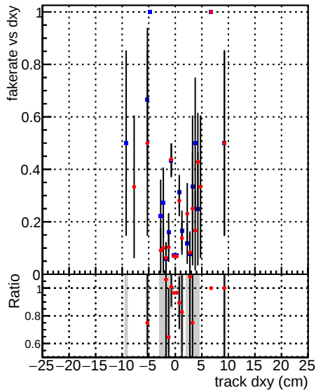
—●— DQM_CKF_TTbase —●— DQM_CKF_TT_retrainOldFiles125_v2_prelimWP_epoch4
