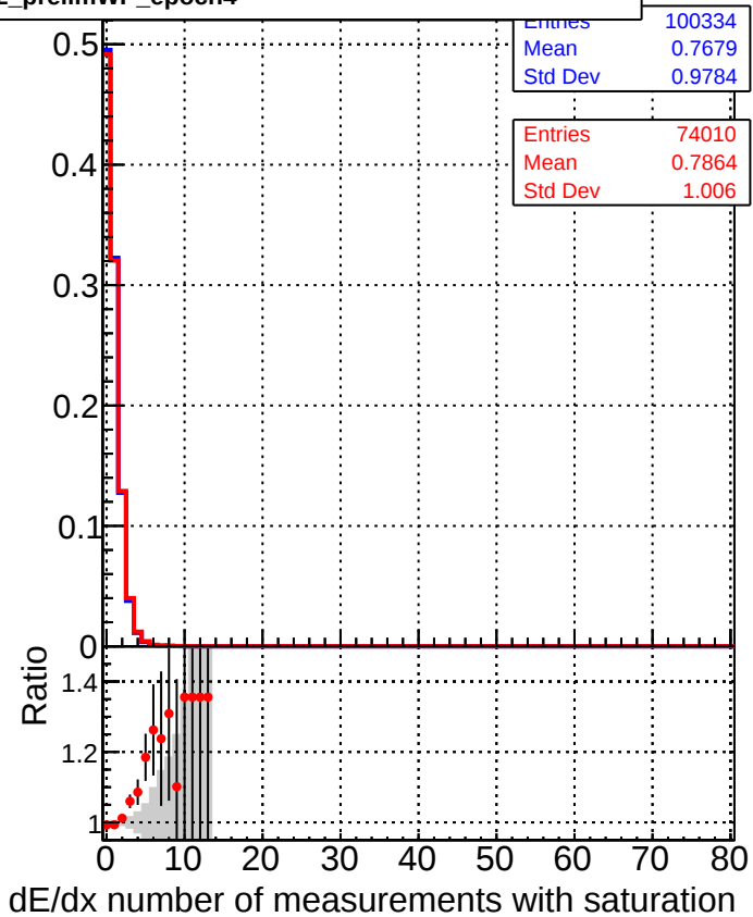
■ DQM_CKF_TTbase ● DQM_CKF_TT_retrainOldFiles125_v2_prelimWP_epoch4
