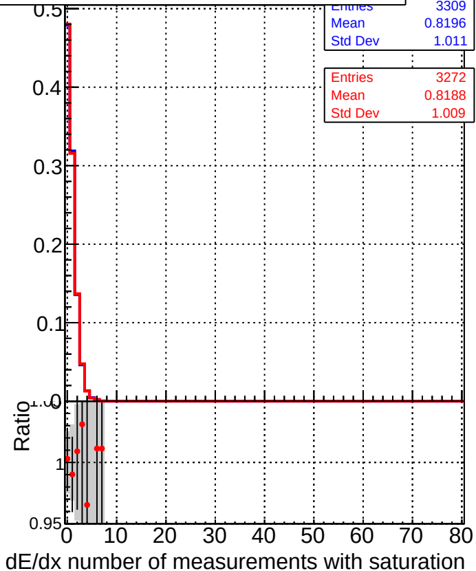
■ DQM_CKF_TTbase ● DQM_CKF_TT_retrainOldFiles125_v2_prelimWP_epoch4
