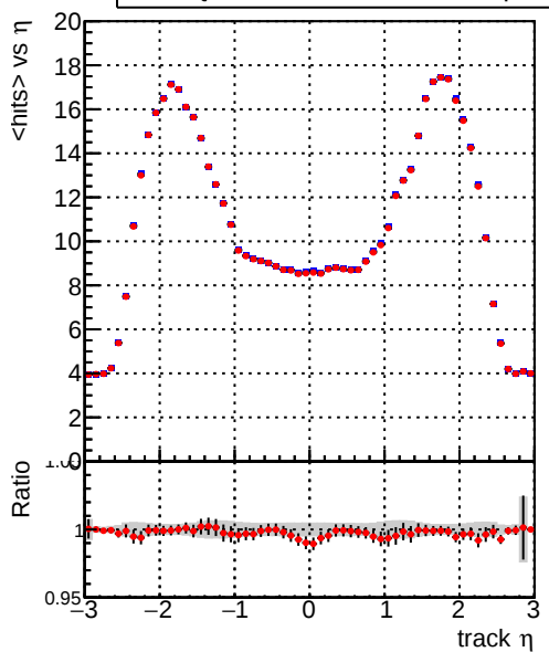
— DQM_CKF_TTbase — DQM_CKF_TT_retrainOldFiles125_v2_prelimWP_epoch4
