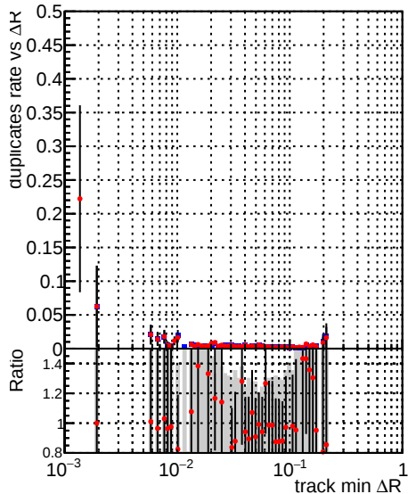
—•— DQM_CKF_TTbase —•— DQM_CKF_TT_retrainOldFiles125_v2_prelimWP_epoch4
