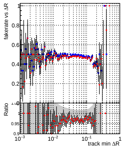
—•— DQM_CKF_TTbase —•— DQM_CKF_TT_retrainOldFiles125_v2_prelimWP_epoch4
