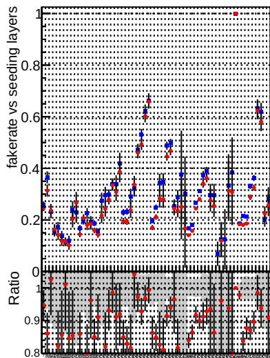
Fake rate vs. ◆ DQM CKF TTbase ● DQM CKF TT_retrainOldFiles125_v2_prelimWP
