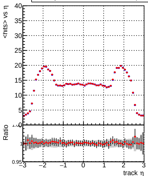
— DQM_CKF_TTbase — DQM_CKF_TT_retrainOldFiles125_v2_prelimWP
