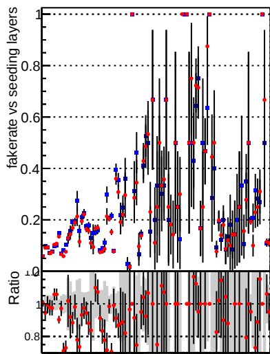
Fake rate vs. —◆— DQM CKF TTbase —★— DQM CKF TT_retrainOldFiles125_v2_prelimWP
