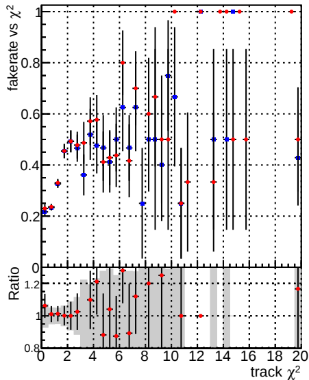
Fake rate vs. —◆— DQM CKF TTbase —◆— DQM CKF TT_retrainOldFiles125_v2_prelimWP
