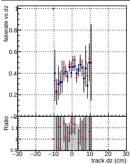
Fake rate vs dz DQM CKF TTbase DQM CKF TT_retrainOldFiles125_v2_prelimWP
