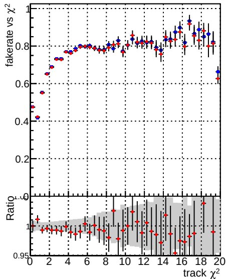
Fake rate vs. \chi^2 Legend: —•— DQM CKF TTbase —•— DQM CKF TT_retrainOldFiles125_v2_prelimWP
