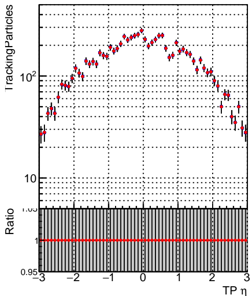
— DQM_CKF_TTbase — DQM_CKF_TT_retrainOldFiles125_v2_prelimWP
