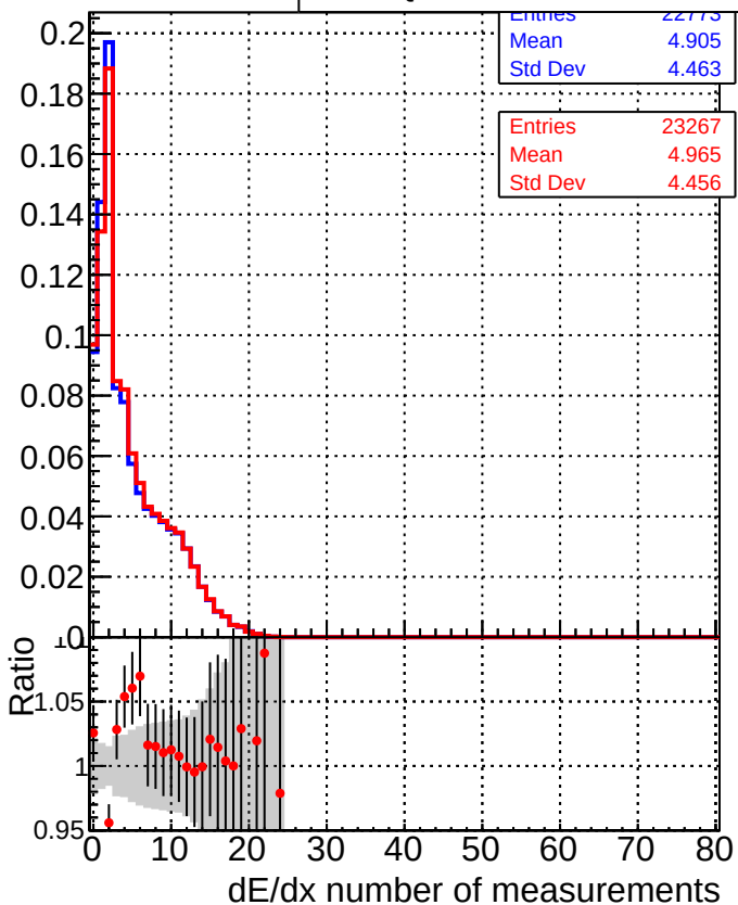
— DQM_CKF_TTbase — DQM_CKF_TT_retrainOldFiles125_v2_prelimWP
