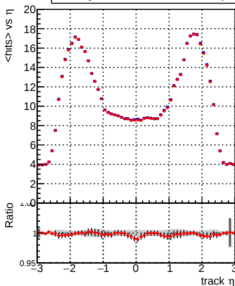
— DQM_CKF_TTbase — DQM_CKF_TT_retrainOldFiles125_v2_prelimWP
