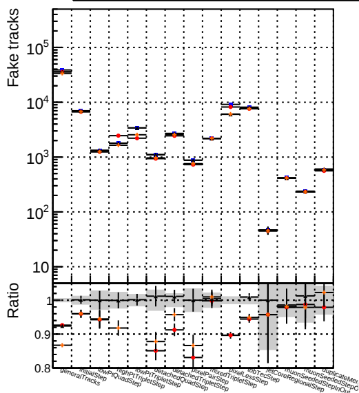
Number ● DQM_mkFit_TT_retrainOldHes125_V2_premHWR_5iter ▲ DQM_mkFit_TT_baseline_6iter ◆ DQM_mkFit_TT RetrainV2_WP1_6iter
