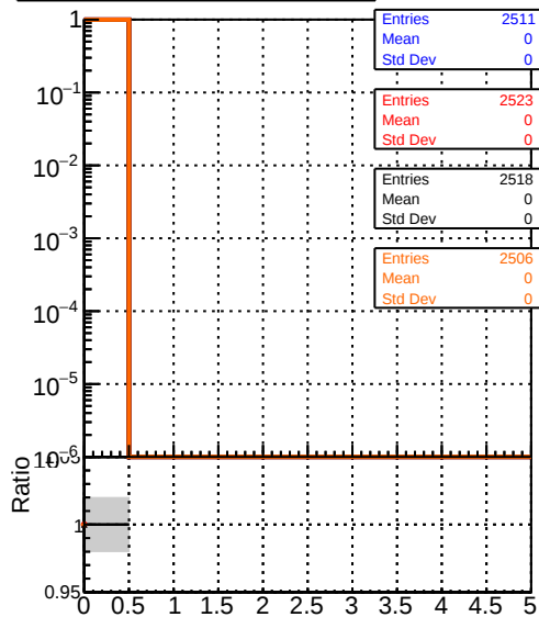
— DQM_mkFit_TTbase — DQM_mkFit_TT_retrainOldFiles125_v2_prelimWP_5iter — DQM_mkFit_TT_baseline_6iter — DQM_mkFit_TT_RetrainV2_WP1_6iter
