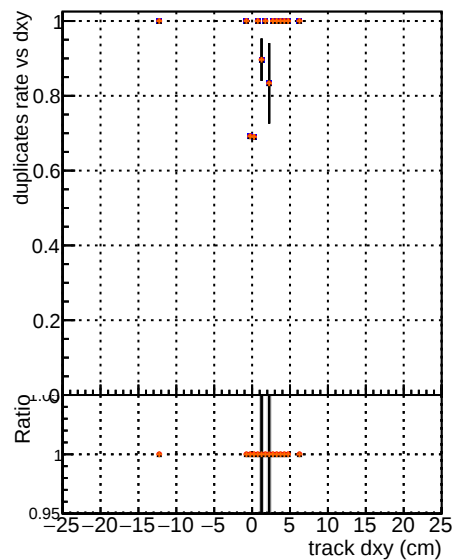
DOM mkFit Tbase RetainOldFiles125 v2 prelimWP_5iter DOM mkFit RetainV2 WP1 6iter
