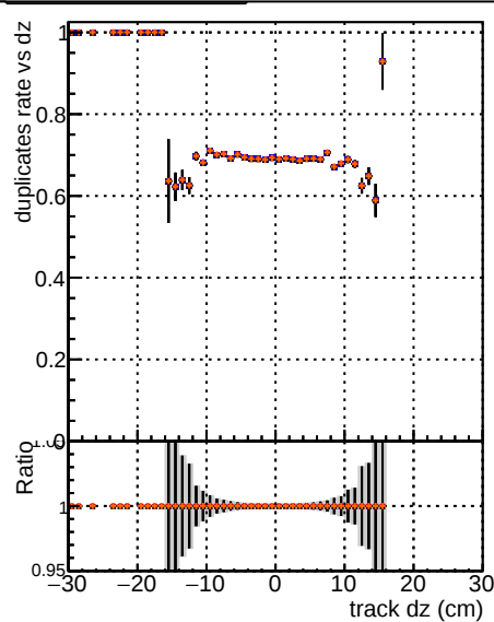
DOM mkFit Tbase RetainOldFiles125 v2 prelimWP_5iter DOM mkFit RetainV2 WP1 6iter
