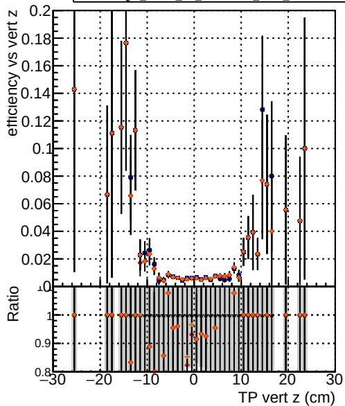
Efficiency vs. sim PV z DOM_mkFit TTbase DOM_mkFit TT_retrainOldFiles125_v2_prelimWP_5iter DOM_mkFit TT_baseline_6iter DOM_mkFit TT_RetrainV2_WP1_6iter
