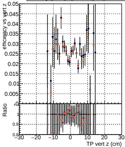
Efficiency vs. TP vert z (cm) —•— DQM_mkFit_TTbase —•— DQM_mkFit_TT_retrainOldFiles125_v2_prelimWP_5iter —•— DQM_mkFit_TT_baseline_6iter —•— DQM_mkFit_TT_RetrainV2_WP1_6iter
