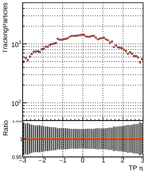
◆ DQM_mkFit_TTbase ◆ DQM_mkFit_TT_retrainOldFiles125_v2_prelimWP_5iter ◆ DQM_mkFit_TT_baseline_6iter ◆ DQM_mkFit_TT_RetrainV2_WP1_6iter
