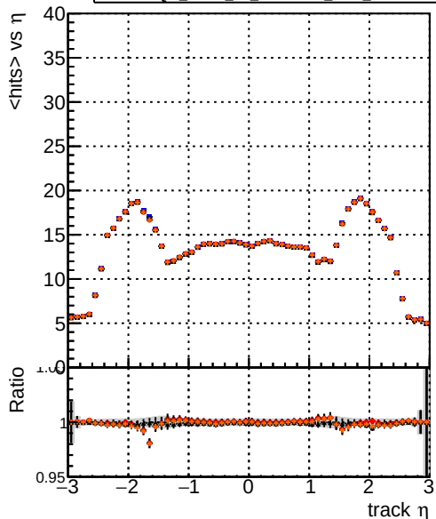
DQM_mkFit_TTbase DQM_mkFit_TT_retrainOldFiles125_v2_prelimWP_5iter DQM_mkFit_TT_baseline_6iter DQM_mkFit_TT_RetrainV2_WP1_6iter mean hit
