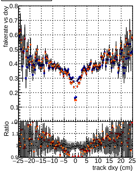
DQM mkFit Ttbase Retrain v2 WP1 6iter
