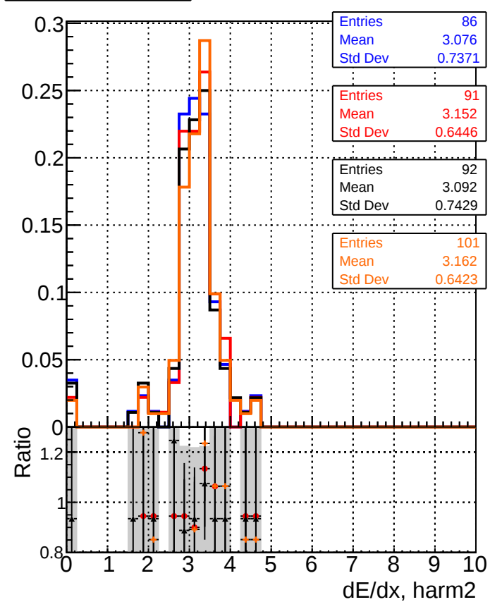
—■— DQM_mkFit_TTbase —●— DQM_mkFit_TT_retrainOldFiles125_v2_prelimWP_5iter —▲— DQM_mkFit_TT_baseline_6iter —◆— DQM_mkFit_TT_RetrainV2_WP1_6iter
