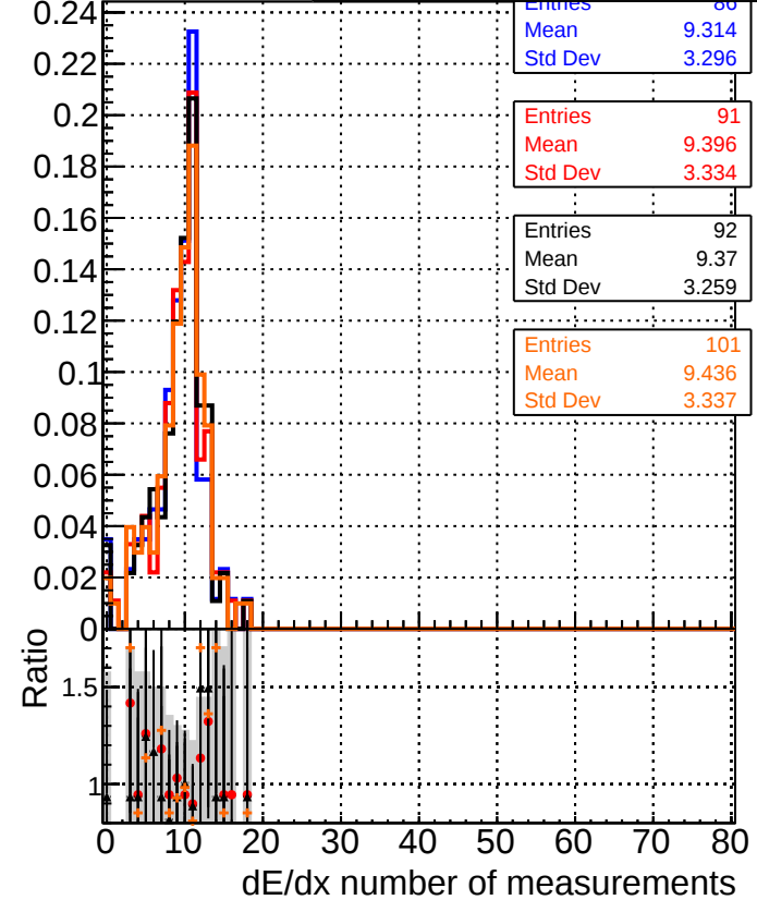
—■— DQM_mkFit_TTbase —●— DQM_mkFit_TT_retrainOldFiles125_v2_prelimWP_5iter —▲— DQM_mkFit_TT_baseline_6iter —◆— DQM_mkFit_TT_RetrainV2_WP1_6iter
