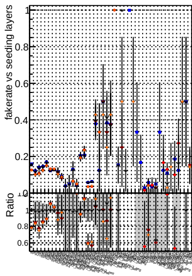
Fake rate vs. DQM mkFit DQM mkFit + Tbase Retrain v2 WP1 6iter
