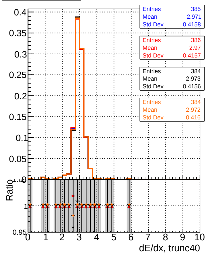
Legend: DQM_mkFit TTbase DQM_mkFit TT_retrainOldFiles125_v2_prelimWP_5iter DQM_mkFit TT_baseline_6iter DQM_mkFit TT_RetrainV2_WP1_6iter
