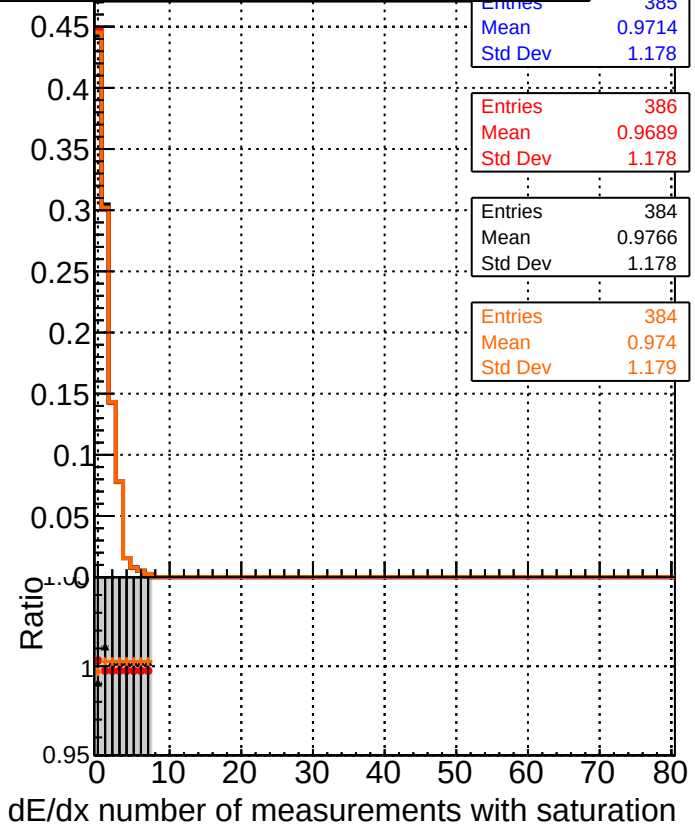
Legend: DQM_mkFit TTbase DQM_mkFit TT_retrainOldFiles125_v2_prelimWP_5iter DQM_mkFit TT_baseline_6iter DQM_mkFit TT_RetrainV2_WP1_6iter
