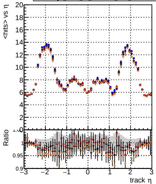
mean hit — DQM_mkFit_TTbase — DQM_mkFit_TT_retrainOldFiles125_v2_prelimWP_5iter — DQM_mkFit_TT_baseline_6iter — DQM_mkFit_TT_RetrainV2_WP1_6iter
