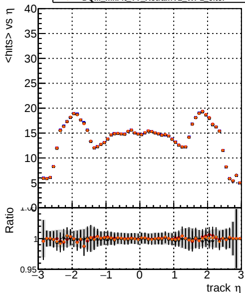
— DQM_mkFit_TTbase — DQM_mkFit_TT_retrainOldFiles125_v2_prelimWP_5iter — DQM_mkFit_TT_baseline_6iter — DQM_mkFit_TT_RetrainV2_WP1_6iter mean hits
