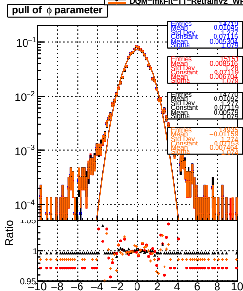
DOM mkFit TTbase RetrainOldFiles125 v2_prelimWP_5iter RetrainNewFiles125 v2_prelimWP_5iter Retrainv2 WP1 6iter
