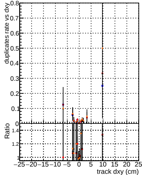
DOM mkFit Tbase DOM mkFit + Tbase RetainOldFiles125 v2 prelimWP_5iter DOM mkFit + Tbase RetainOldFiles125 v2 prelimWP_6iter
