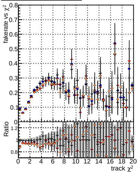
Fake rate vs. DQM mkFit TTbase DataTrainOldFiles125 v2 prelimWP_5iter DataTrainv2 WP1 6iter
