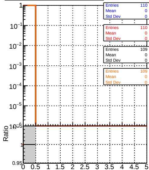
mean hit — DQM_mkFit_TTbase — DQM_mkFit_TT_retrainOldFiles125_v2_prelimWP_5iter — DQM_mkFit_TT_baseline_6iter — DQM_mkFit_TT_RetrainV2_WP1_6iter
