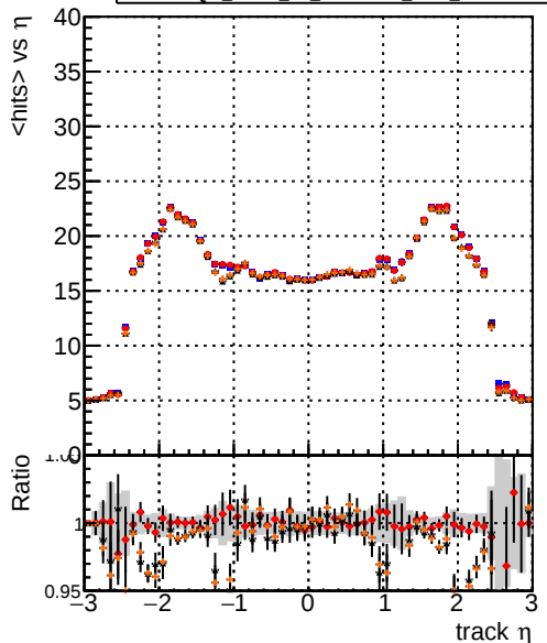
mean hits vs \eta DQM_mkFit_TTbase DQM_mkFit_TT_retrainOldFiles125_v2_prelimWP_5iter DQM_mkFit_TT_baseline_6iter DQM_mkFit_TT_RetrainV2_WP1_6iter
